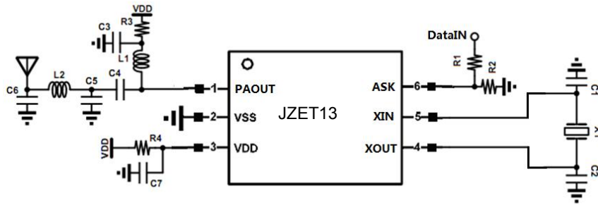
图3: JZET13应用电路
