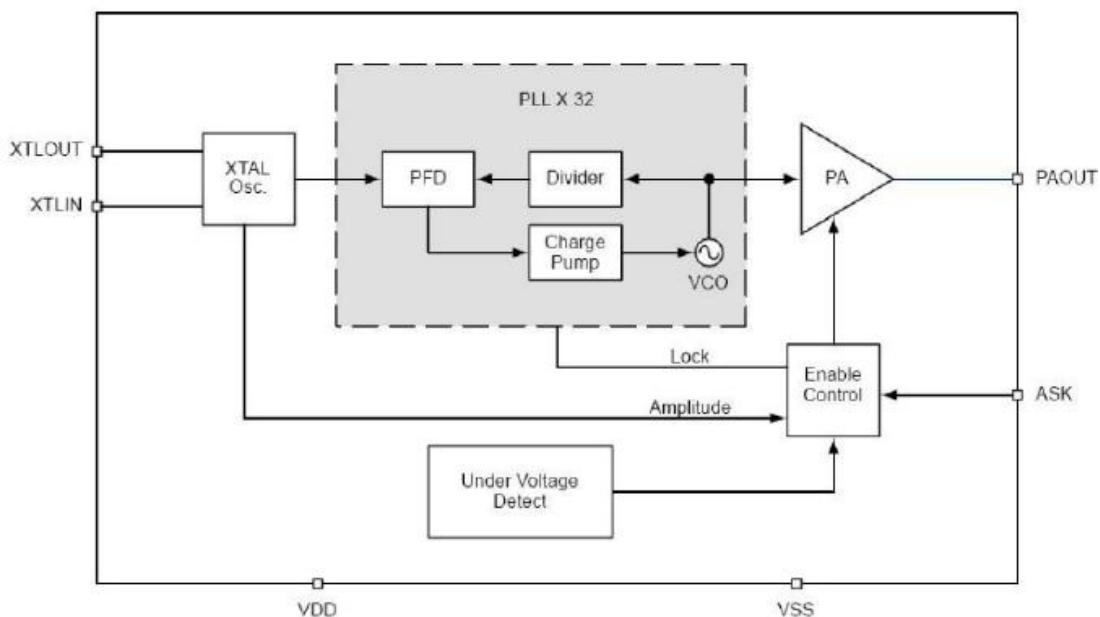
图1: 芯片框图
