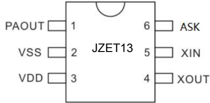
图2: JZET13 芯片脚位图
