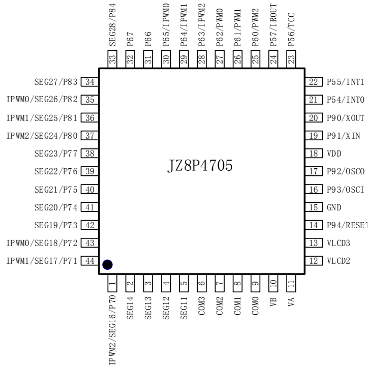
JZ8P4705-44PIN 脚位图
