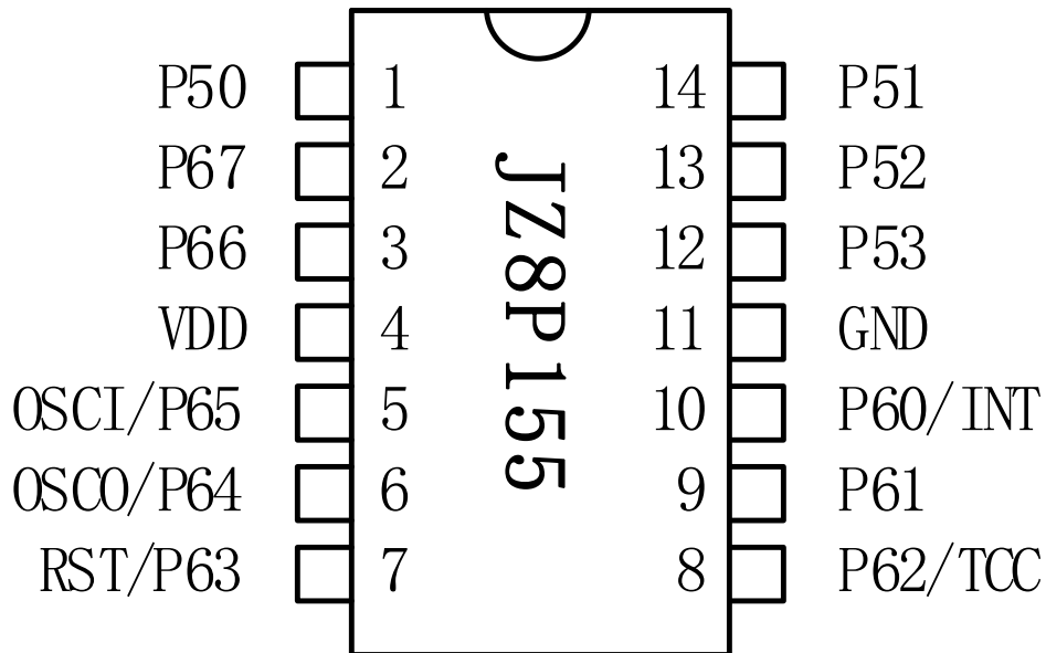
JZ8P155-14PIN 脚位图
