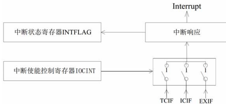
中断说明图
