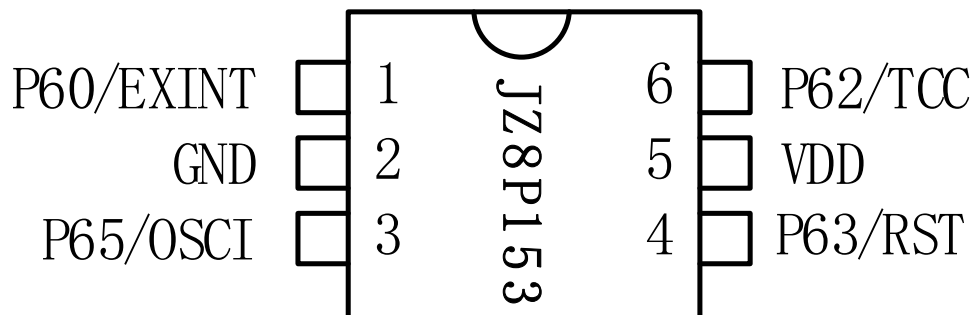
JZ8P153-6PIN 脚位图
