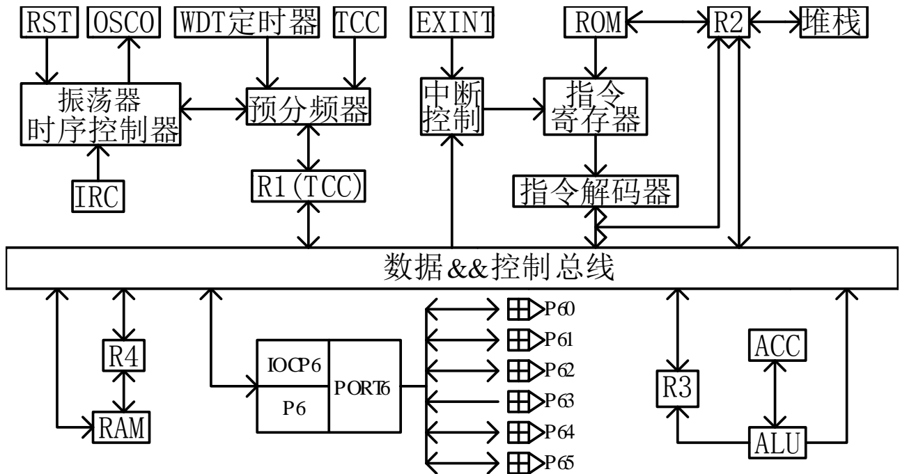
JZ8P153 功能框图
