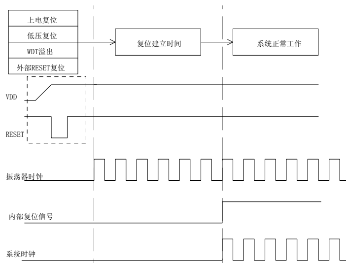
复位功能原理图
