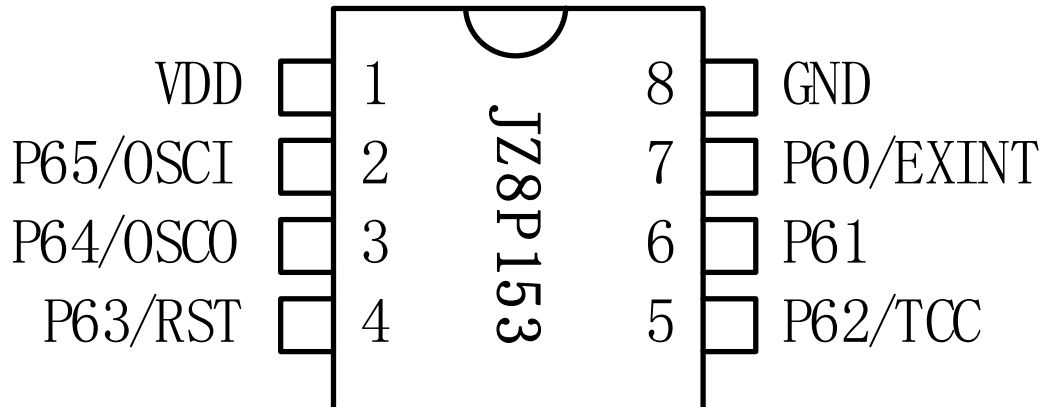
JZ8P153-8PIN 脚位图
